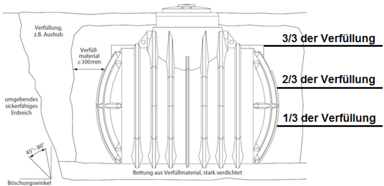
Abbildung 4: Ausführung des Einbaus anhand eines Premium 4000 L Erdtanks mit Tankabdeckung Basic
